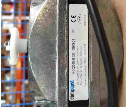
Q-motor
